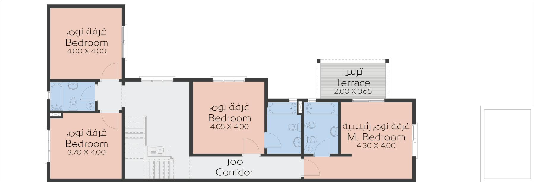
مسقط الدور الأول First Floor Plan
